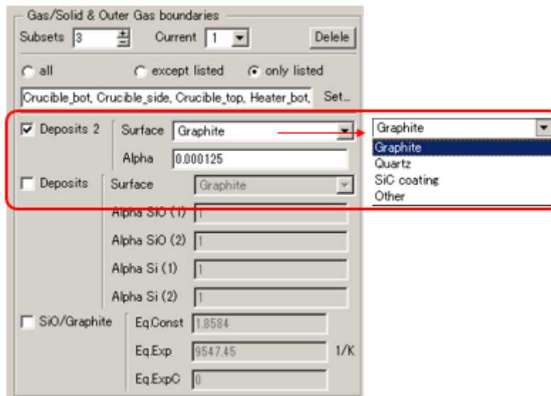
図 3. ガス/固体境界の設定画面(Deposits2)
